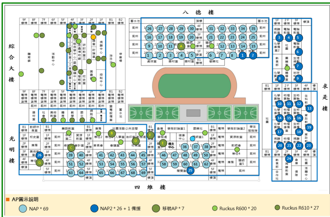
臺北市成功高級中學-109前瞻計畫無線AP建置示意圖
